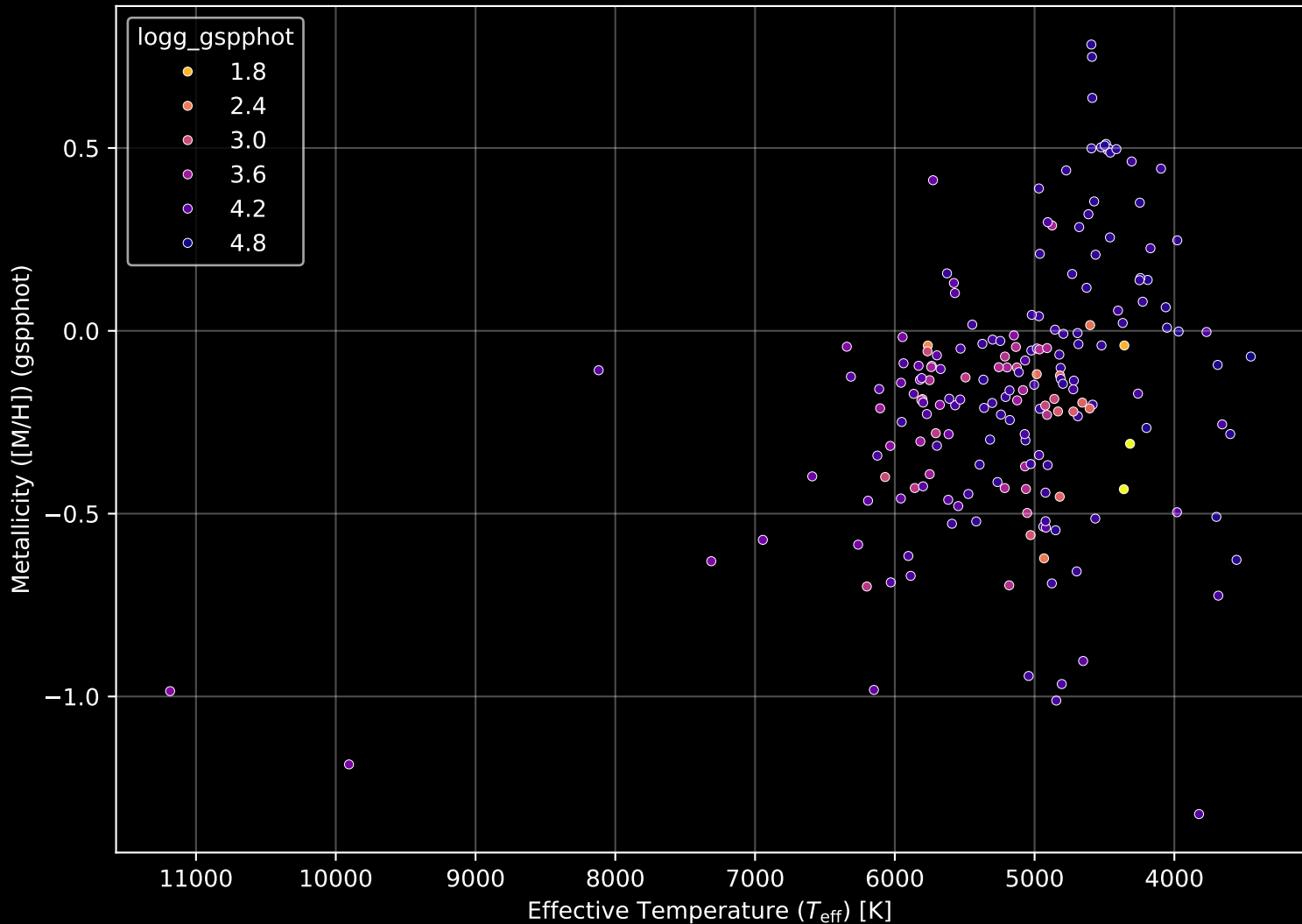
APOGEE DR17 Field: [099+56_btx] Stellar Population Parameters (n= 194)
